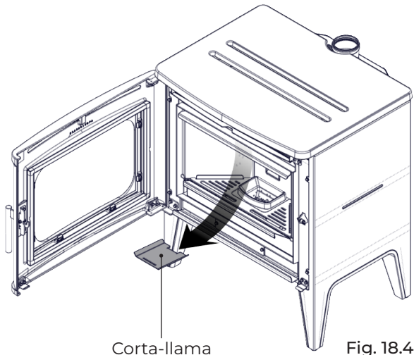
Corta-llama Fig. 18.4
