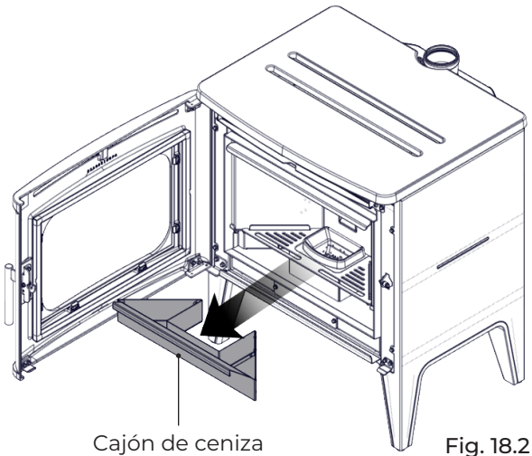
Cajón de ceniza Fig. 18.2
