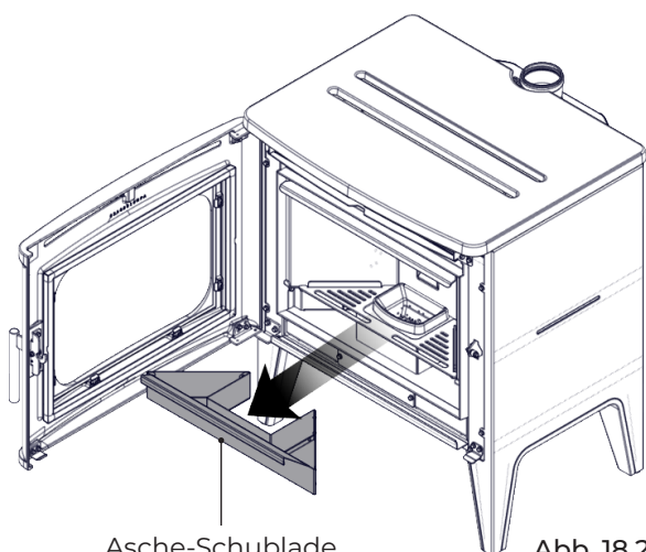
Asche-Schublade
