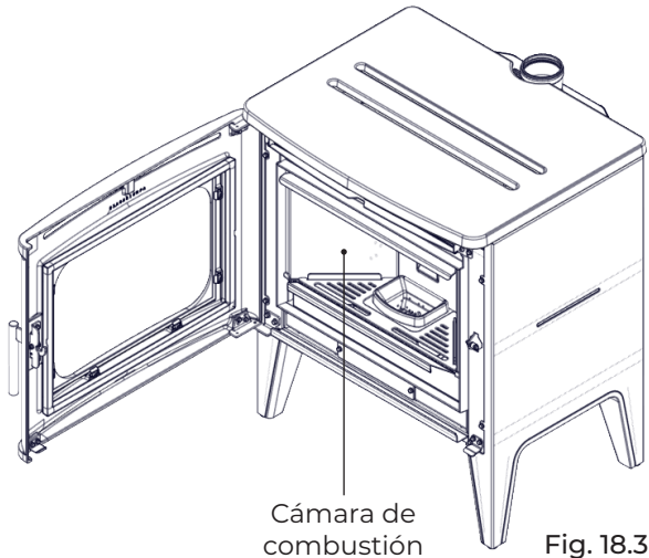
Cámara de combustión Fig. 18.3
