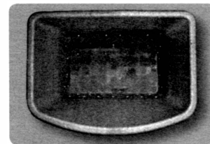
Cestello che necessita di pulizia con i fori otturati dalla cenere
